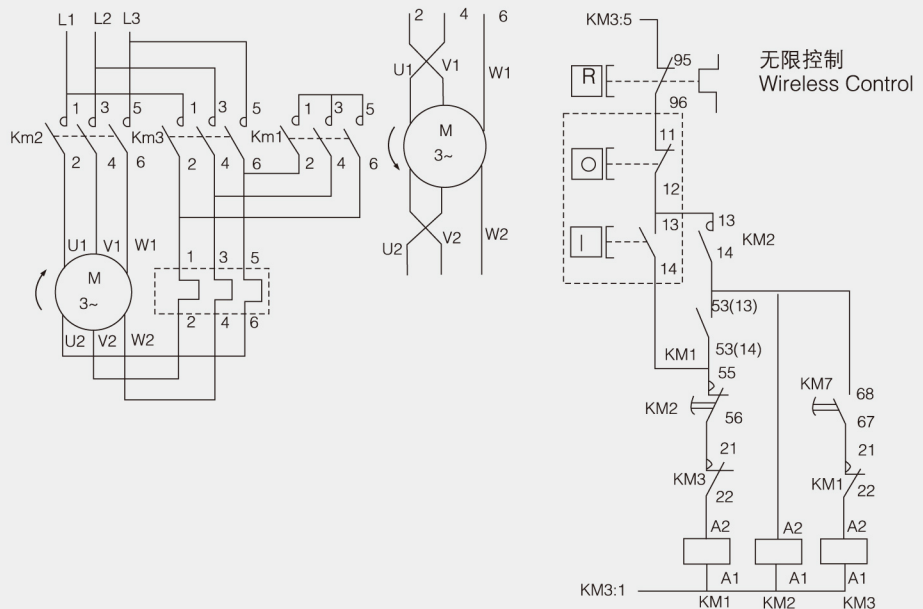
电路图 Wiring Diagram
